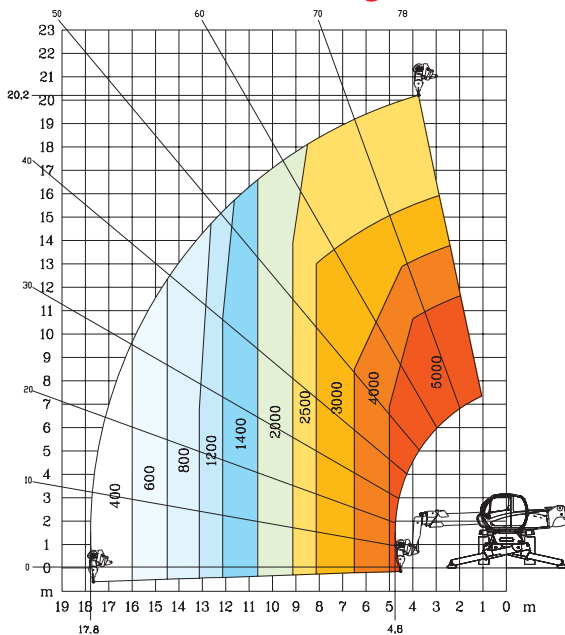
Rotation sur stabilisateurs déployés avec nacelle 365/1000 kg
